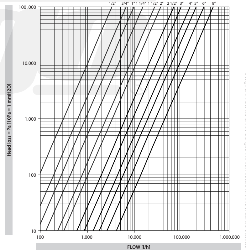
DRUCKVERLUSTDIAGRAMM / HEAD LOSS DIAGRAM
