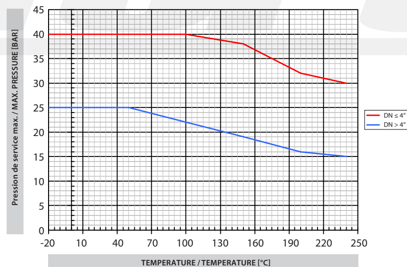
Diagramme Pression-Température / PRESSURE TEMPERATURE DIAGRAM
