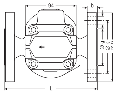
UNA 14h / UNA 16h, flanged design
