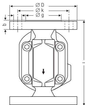
UNA 14h / UNA 16v, flanged design
